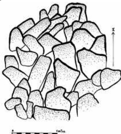
FIG. 3.—ARROLAMENDI II. Planta en la zanja W.
